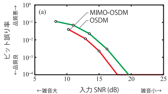
図 3：マルチチャネル OSDM と MIMO に対応したマルチチャネル OSDM の性能 (発表論文②より)
