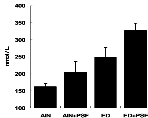
図1 食物繊維の摂取が腸管透過性に及ぼす影響の解析
