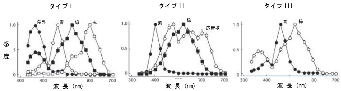
図 1. 3 タイプの個眼に含まれる視細胞の分光感度
