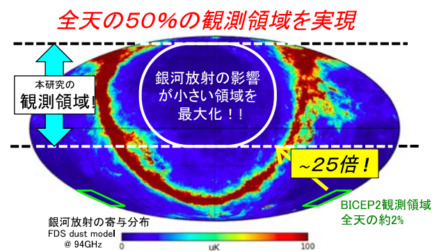
図 1. 本研究でカバーする観測領域
