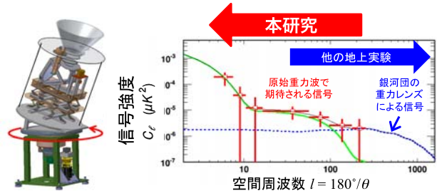
図 2. GroundBIRD 望遠鏡と 3 年間の観測で期待される空間スペクトル
