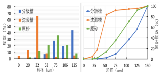
図 3 粒度度数分布 傾斜角度 60 度、流量 40L/min
