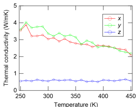
図4 結晶構造モデルのスマネンにおける格子熱伝導率の方向依存性
