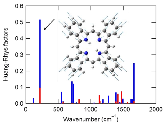
図3 BP における Huang-Rhys 因子の振動数依存性に対応する基準振動モード (赤色は中性-正荷電状態間、青色は中性-負荷電状態間を表す)
