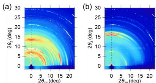
図2 (a) BP および(b) PDI 薄膜の GIXD パターン
