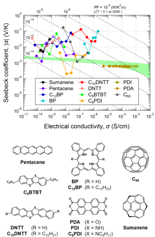
図 1 各分子におけるゼーベック係数と導電率の関係 (右側のプロットほど高温での測定を表し、●は n 型、○は p 型のゼーベック係数を表す)
