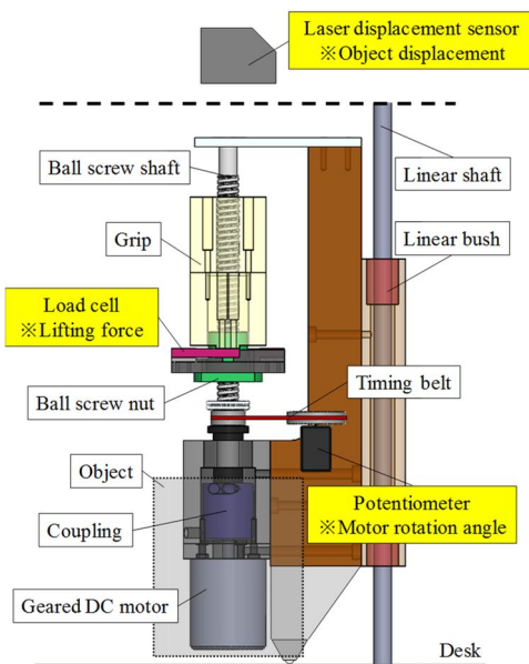
図 8 実験装置の概要
