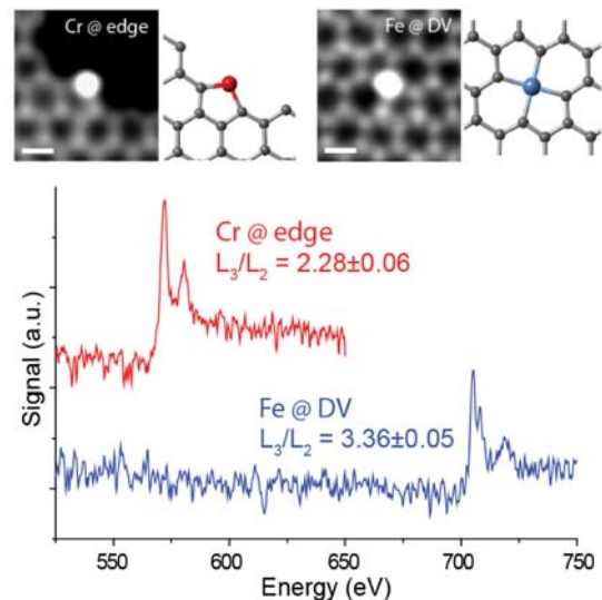
図 単原子のスピン状態測定の予備実験例。L吸収端における枝分かれ比(L 3 /L 2 )は、注目する3d遷移金属のdサブバンド内の電荷移動量を反映しており、グラフエッジ上のCr原子も、複空孔(DV)中のFe原子も高スピン状態であることがわかる。
