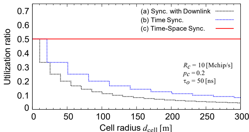
図1 チャネル利用効率の数値計算例
