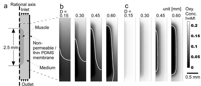
図2 マイクロ流体デバイスで筋組織を培養した場合の酸素濃度分布。(a)解析モデル、(b)壁面からの酸素供給が無い場合、(c)壁面から酸素供給がある場合。
