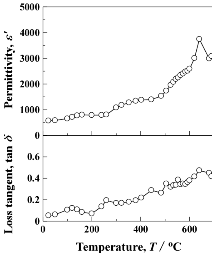
図4 電気泳動堆積法により \text{BaTi}_2\text{O}_5 粒子膜を形成させた後に、 \text{BaTiO}_3 前駆体溶液をスピンコートして作製した \text{BaTi}_2\text{O}_5 - \text{BaTiO}_3 コンポジット薄膜の誘電率と誘電正接の温度依存性．分散媒にはエタノール、分散剤にはポリエチレンジアミン (PEI) を用いた．
