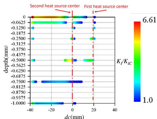
図 12 熱源中心からの距離と深さにおけるき裂開口領域
