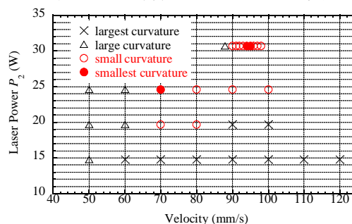
図 13 走査速度と 2 点目のレーザー出力における加工成立領域
