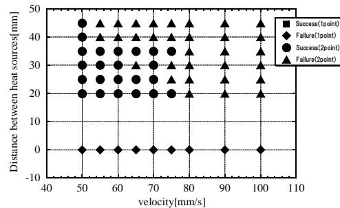
図 8 走査速度と2点間距離における加工成立領域 ( t=1.0\text{ mm} )
