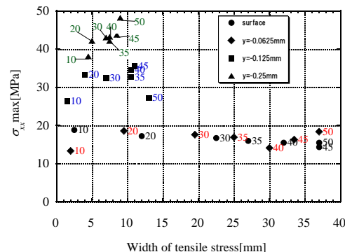
図7 深さ毎の引張応力場 \sigma_{xx} の長さ最大引張り応力
