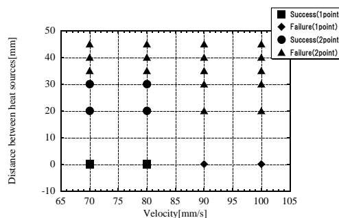
図 10 走査速度と2点間距離における加工成立領域 ( t=0.5\text{ mm} )
