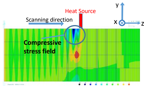
図5 複数走査実験における応力 \sigma_{yy} 分布
