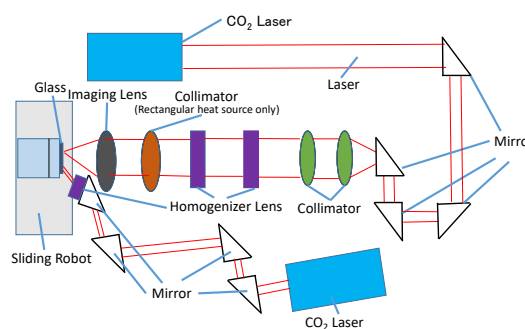
図3 実験装置概略図
