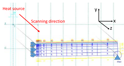
図4 FEM 解析モデル
