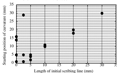
図 15 初期き裂長さと反りの起点位置との関係
