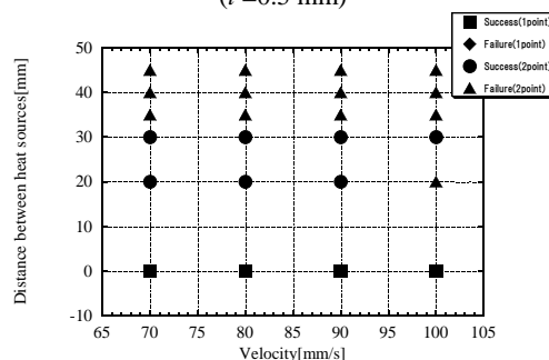
図 11 走査速度と2点間距離における加工成立領域 ( t=0.3\text{ mm} )
