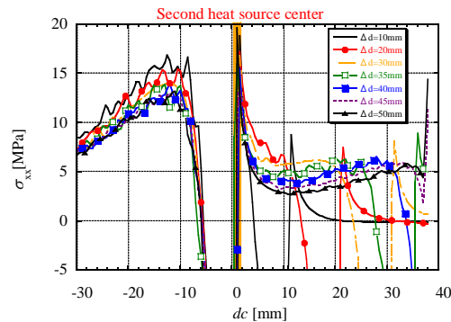
図6 \Delta d 毎の引張応力と熱源位置からの距離 d_c の関係 ( y=0, \Delta d=10, 20, 30, 35, 40, 45, 50\text{ mm} )
