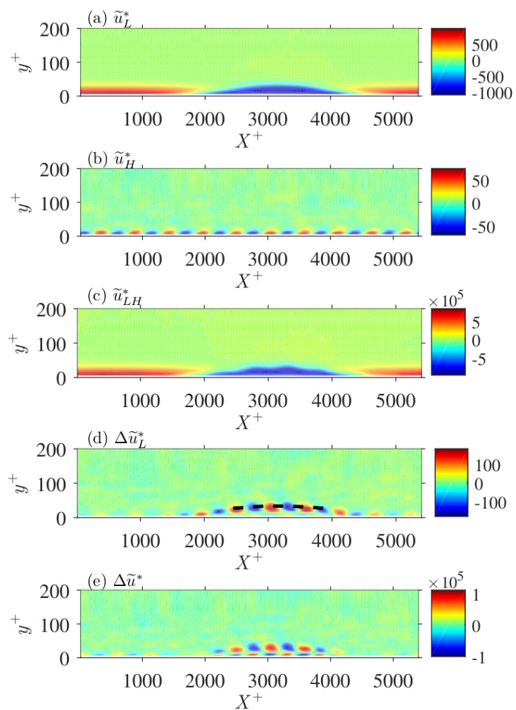
図1 励起された乱れ構造の等値線図
