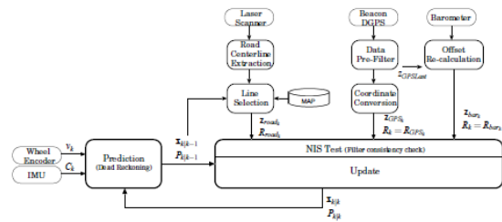
図 7 計測系のブロック線図
