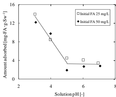
図 5 フルボ酸のシュベルトマナイトへの吸着の pH の影響
