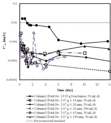
図2 山土不溶化土壌の下にバリア層を設置した場合のヒ素流出濃度
