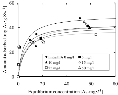
図 4 フルボ酸濃度のヒ素吸着量への影響
