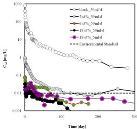
図1 山土に 947mg-As/kg-soil 添加した模擬汚染土壌に対するシュベルトマナイトの不溶化の効果
