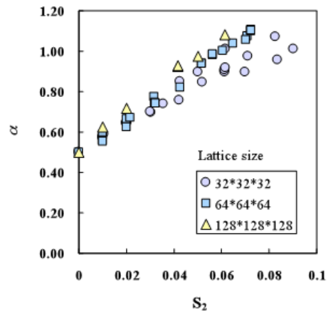
図 7 第 2 相割合 S_2 とべき乗指数 \alpha との関係
