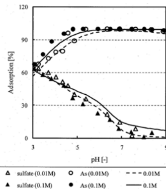
図3 回分吸着実験とモデルとの比較
