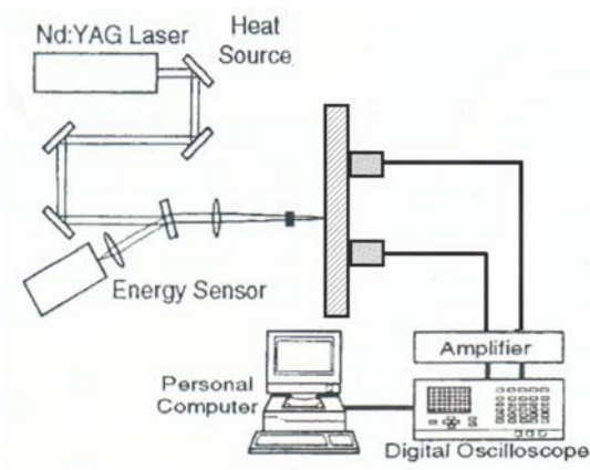
レーザ熱衝撃実験装置
