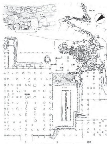
図-2 義景館跡庭園平面図・立面図
