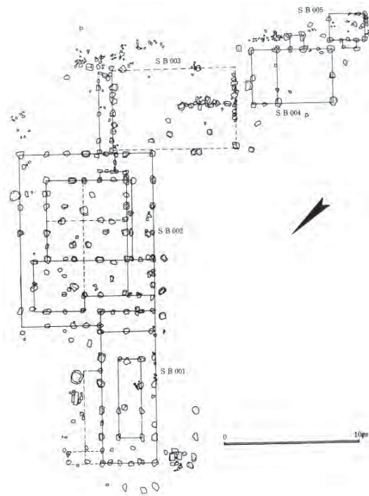
礎石建物実測図
