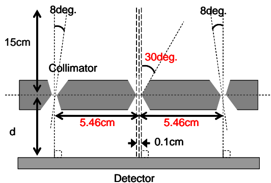
図7 ピンホールの断面図
