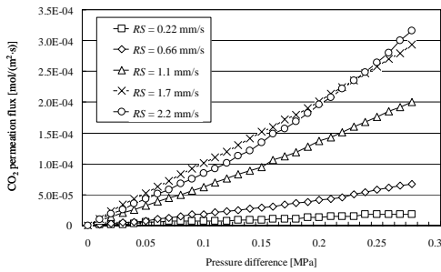
図7 TiO 2 膜コーティング済み多孔質体気体分離膜前後の差圧とCO 2 透過流束との関係 (バッチ式)
