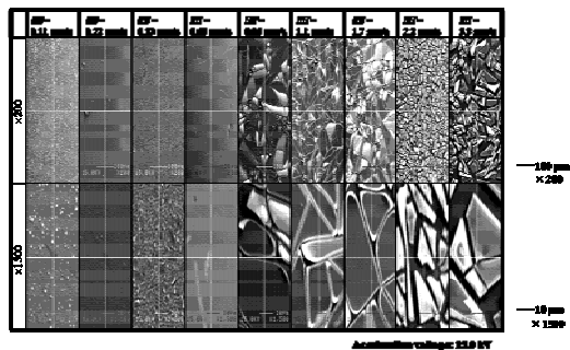
図3 異なる RS 条件でのTiO 2 膜のSEM写真
