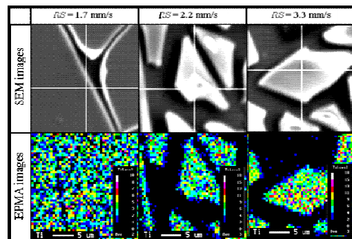
図5 異なる RS 条件でのTiO 2 膜のSEM写真とEPMA分析結果 ( RS :1.7、2.2、3.3mm/s)
