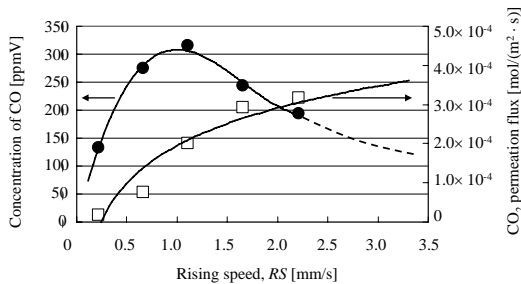
図8 CO濃度とCO 2 透過流束の比較
