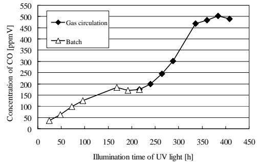
図9 CO濃度経時変化 (バッチ式→ガス循環式)
