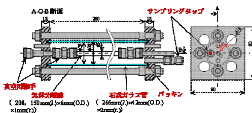
図1 光触媒リアクター概要
