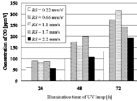
図6 CO濃度経時変化の比較 (バッチ式)
