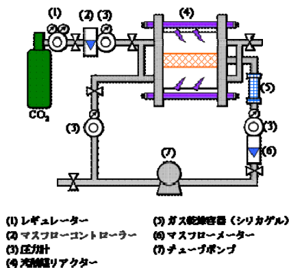
図2 実験装置外略図
