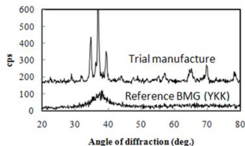
図 6 試作合金の X 線回折像
