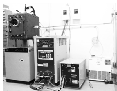
図 3 作製完了した溶解アーク炉外観
