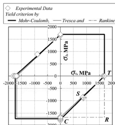
図 8 \text{Zr}_{55}\text{Cu}_{30}\text{Al}_{10}\text{Ni}_5 BMG の破損曲面(常温)
