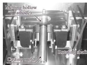
図 4 銅製ハース部および鑄型外観
