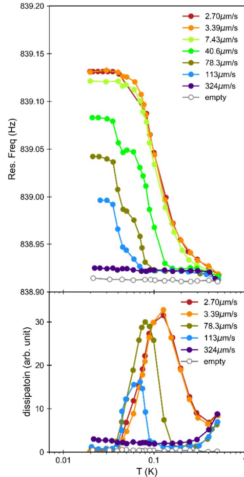
図3:(上段)固体ヘリウム共鳴周波数の温度依存性。(下段)振動子内の固体ヘリウムエネルギー散逸の温度依存性。散逸データは特徴的な変化の見られる振動速度のデータのみ掲載。
