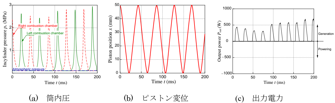
図6 断続的速度制御適用時の解析結果
