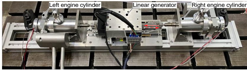
図4 デュアルシリンダ FPEG 実験の外観
