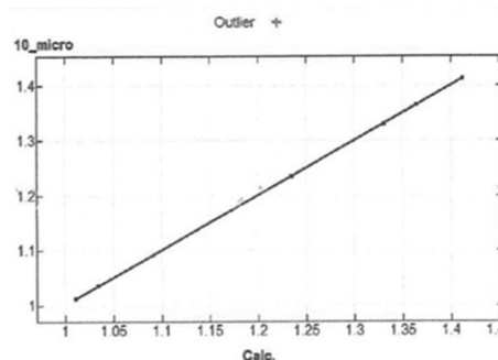
図 6. 化学構造式とシグナル活性の相関グラフの 1 例。
