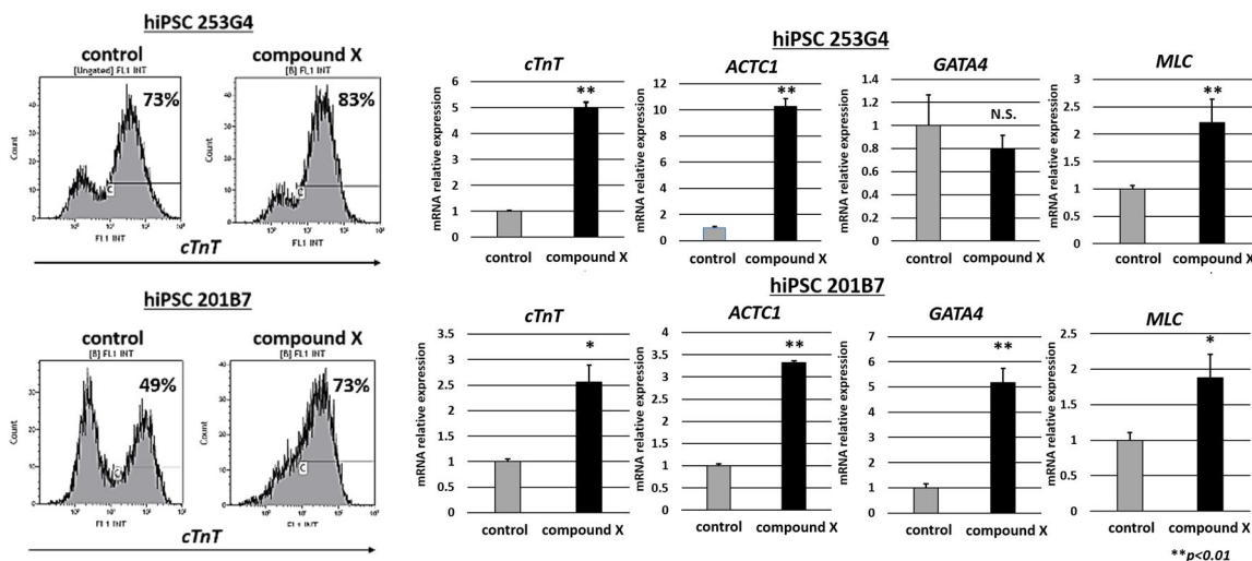
図 5. 同定した化合物添加により、心筋分化効率の改善が FACS、RT-PCR、免疫染色で確認された。
