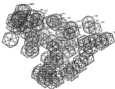
図 3. 標的ドメインからの Ph4 の予測の 1 例。
