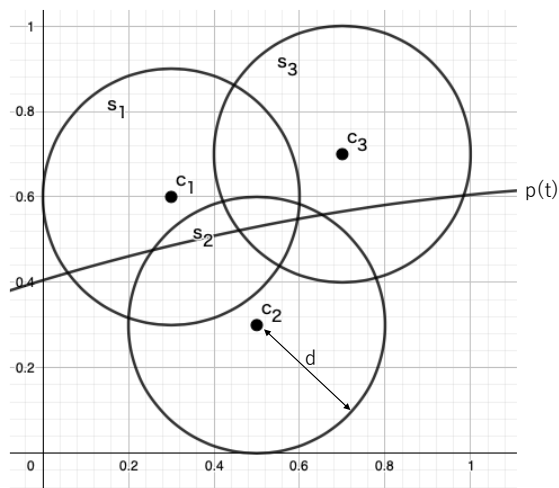
図1. センサの位置関係と人の移動経路
