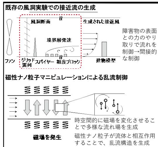
図1. 本研究が目指す新たな乱流制御
