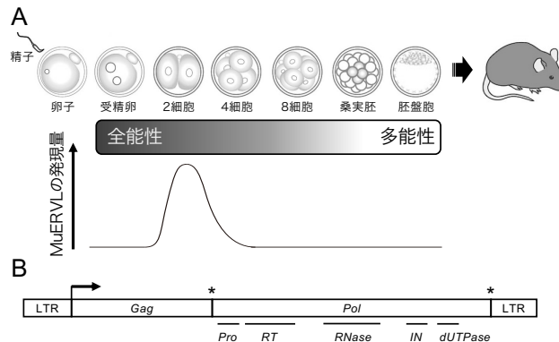
図1. マウス2細胞期胚に一過的に発現するMuERVL A. 2細胞期で起こるゲノムの初期化と同調したMuERVLの活性化と、全能性から多能性への移行を模式的に示す。 B. MuERVLの構造(基準配列 No. Y12713, 6471 bp) LTR: long terminal repeat, Gag: 構造タンパク質, Pol: ウイルス酵素群, Pro: プロテアーゼ, RT: 逆転写酵素, IN: インテグラーゼ, アスタリスクは終止コドン。
