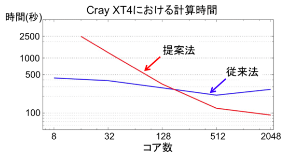
図 3. 演算コア数による計算時間の変化
