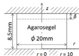
図 2 試料寸法
