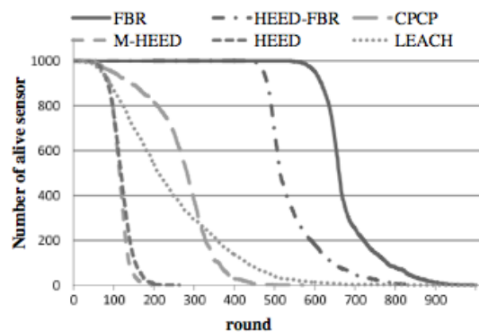
図2 無線センサーの寿命
