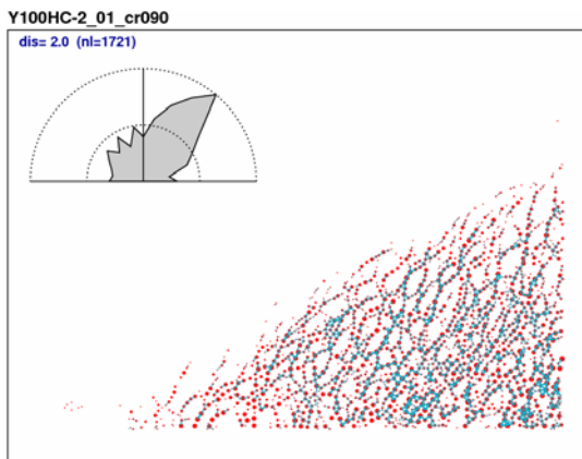
図6 近接する円を結んで描いた応力鎖(青色)と、そのローズダイアグラム(左上インレット)。
