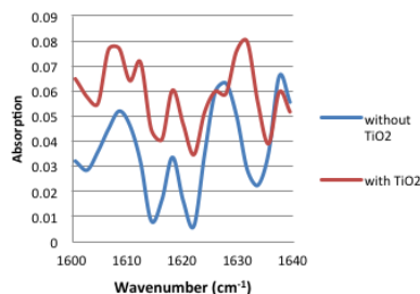
図1 近赤外吸収スペクトル
