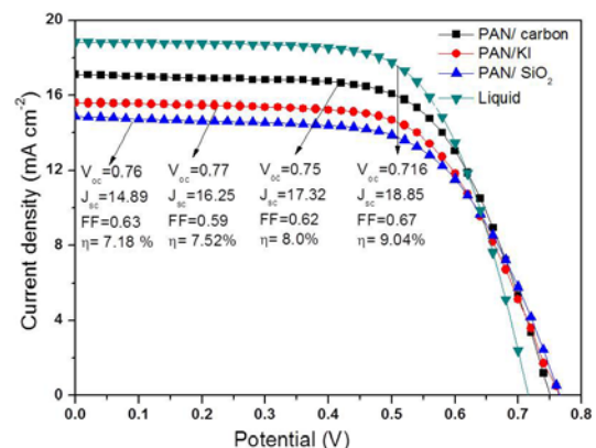
図3 ゲル状高分子電解質と液体電解質を利用した太陽電池のI-V特性
