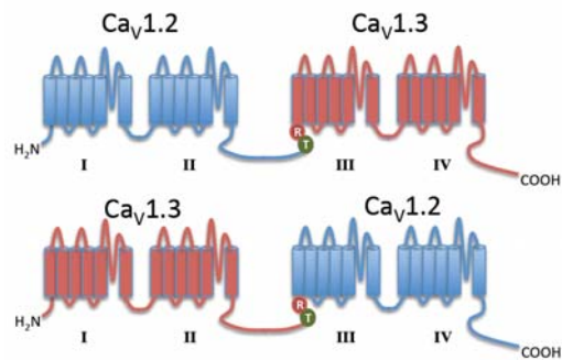
図 1. \text{Ca}_v1.2/\text{Ca}_v1.3 キメラチャネル いずれも HEK 細胞に発現すると \text{Ca}^{2+} 選択性が高く、不活性化の速い電流を構成し、 I_{st} のような持続性 \text{Na}^+ 電流は構成しなかった。
