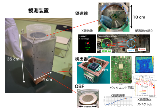
図3：観測装置の性能実証モデル。
