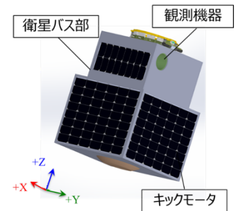
図2：GEO-X衛星。
