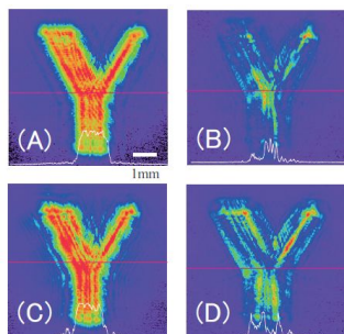
Fig.6 結合画像共振器を伝播した 2次元画像を観測した実験結果
