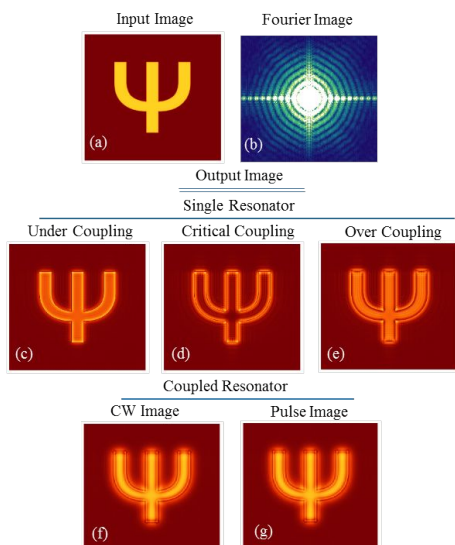
Fig.1 画像共振器の概念図
