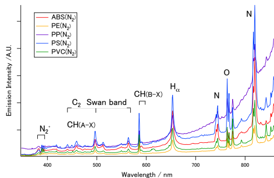
図 6 プラスチックのプラズマ発光スペクトル
