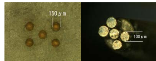
(b) 円形穴—ピン形電極
