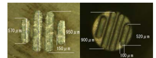
(e) スリットフィン3形電極
