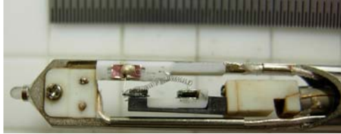
図 3. 小型ヒータを装着したペンシル型 SPM.
