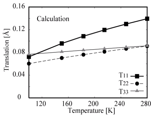
図1 (上図) ペンタセン結晶構造。(中図) ペンタセン分子の並進運動 T11, T22, T33、回転運動 L11, L22, L33。(下図) 熱揺らぎにおける並進運動 T11, T22, T33 の第一原理計算。
