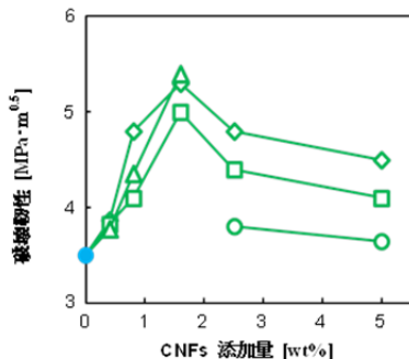
図 5 (△) 1300°C, (◇) 1375°C, (□) 1450°C, (○) 1525°C で PAS した複合体の破壊靱性と CNFs 添加量の関係, (●)アルミナ単体
