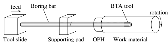
図3 解析モデル
