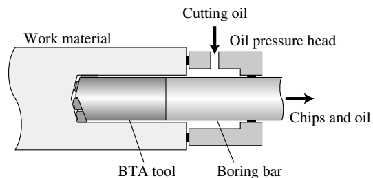
図2 BTA 深穴加工
