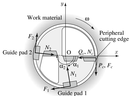
図4 工具先端に作用する力
