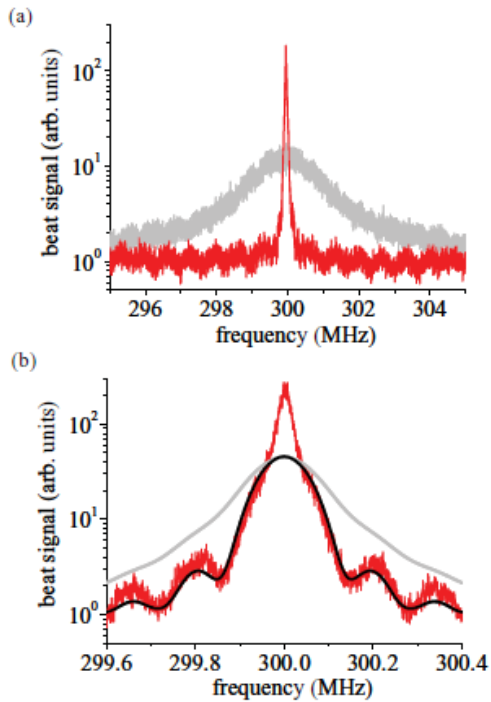
図4 (a)Rb 原子気体の偏光分光信号により線幅狭窄化された DFB レーザーの自己遅延ヘテロダインスペクトル。(b)中心部分のより詳細なスペクトル。
