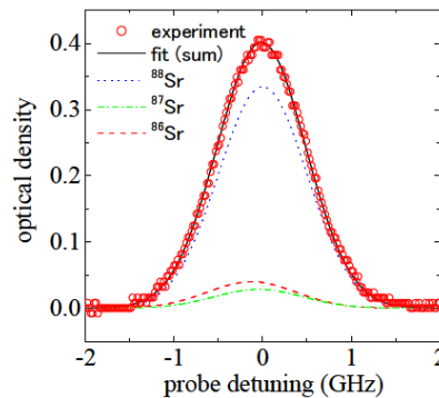
図6 ホローカソードランプ中における Sr 原子気体の線形吸収スペクトル。
