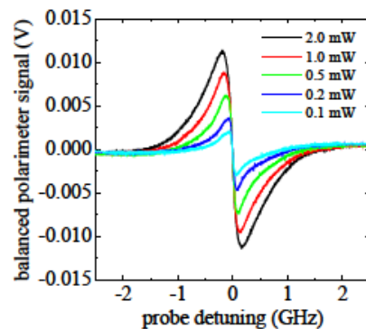
図7 ホローカソードランプ中における Sr 原子気体の偏光分光スペクトル。
