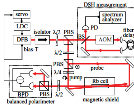
図1 Rb原子気体の偏光分光
