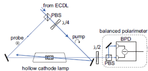
図3 Sr原子気体の偏光分光
