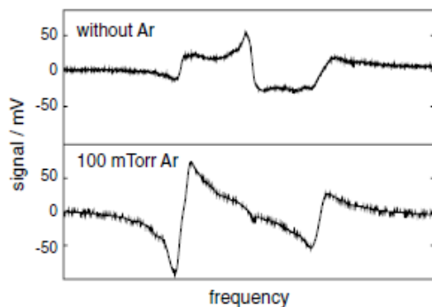
図5 Li6 原子気体の偏光分光信号。左から冷却遷移、クロスオーバー遷移、リポンプ遷移。Ar バッファーガスの導入により、冷却およびリポンプ遷移の信号は増強し、クロスオーバー遷移の信号は減少する。
