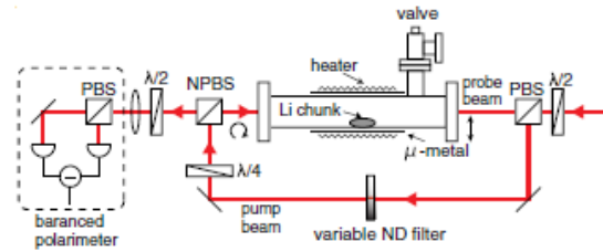
図2 Li6原子気体の偏光分光
