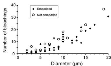
図 2. CLSM によるゲル包埋巨大リポソーム膜(rhodamine-DOPE 染色)の完全消光までのレーザー照射回数。膜上の一点のみに照射し、全体の蛍光が消えるまでの照射回数が粒径に依存し、かつ、包埋と浮遊とで差が無い
