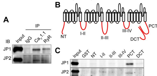
図4 LTCC と JP の結合。A, Ca v 1.1, RyR と JP の共免疫沈降。Ca v 1.1 および RyR の抗体を用いて免疫沈降を行い、JP に対する抗体でウェスタンブロッティングを行った。B, Ca v 1.1 サブユニットの模式図。NT: N 末端, PCT: 近位 C 末端, DCT: 遠位 C 末端。C, Ca v 1.1 の細胞内領域のリコンビナントタンパク質を用いた GST プルダウン。
