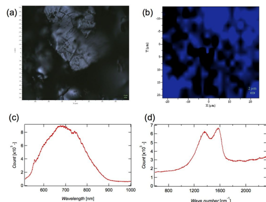
図2: 粗生成物のラマン顕微鏡観察。(a)反射像、(b)発光のマッピング、(c)発光部分における発光スペクトル、(d)非発光部分におけるラマンスペクトル。
