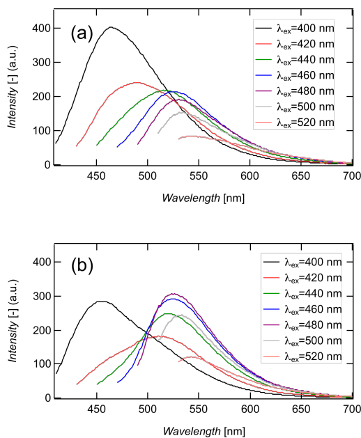
図6：反応温度 550 のカーボンドットの発光スペクトル。送液流量は(a)20 μL/min、(b) 2 μL/min である。
