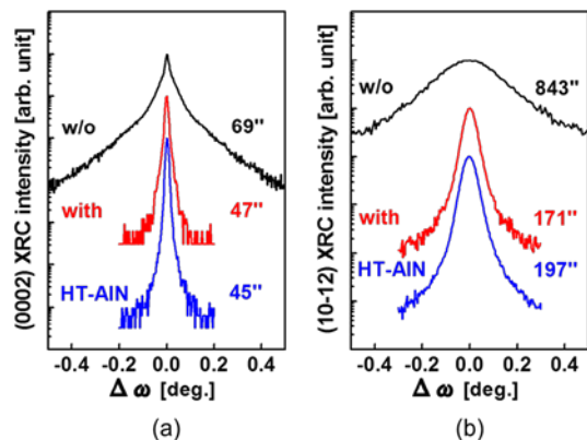
図 1 AlN 緩衝層アニール後及び AlN 2 μm 成長後の(0002)回折と(10-12)回折の X 線ロックンングカーブ
