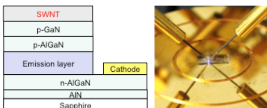
図 2 CNT 電極深紫外 LED の素子構造と発光動作時の写真。
