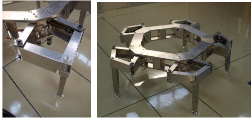
(a) 脚機構 (b) ロボット全体 図4 実スケールの試作ロボット
