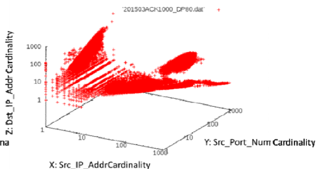
図6: 異なり数解析結果(ACK フィルタ実施)
