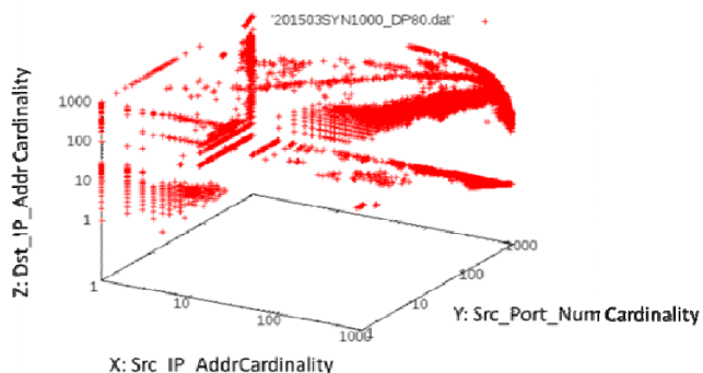
図5: 異なり数解析結果(SYN フィルタ実施)
