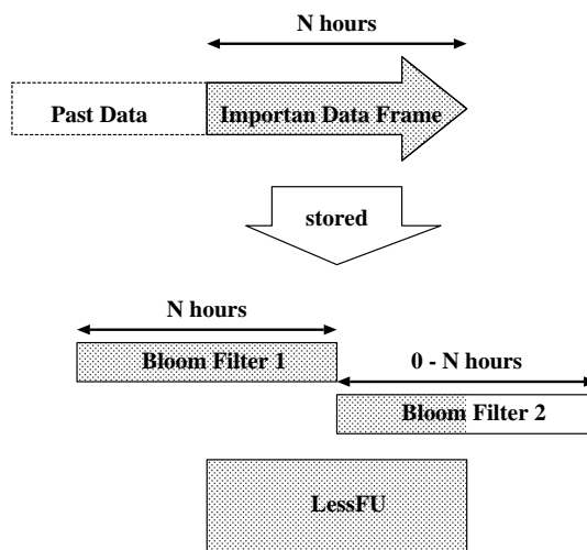
図1: LessFU と Bloom Filter によるメモリ管理
