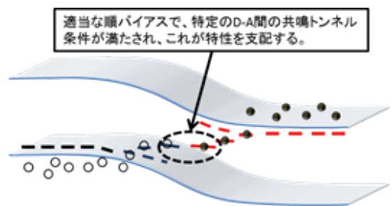
図2. Si ナノ p n ダイオードにおける接合部フロントのドナー・アクセプター間共鳴電子トンネルを示す概念的バンド図。
