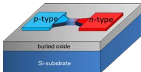
図1. SOI 基板を用いた Si ナノ p n ダイオードの模式図。p n 接合部の厚さ t \approx 10 nm、幅 W \approx 10 nm、長さ L = 50-100 nm 程度とする。
