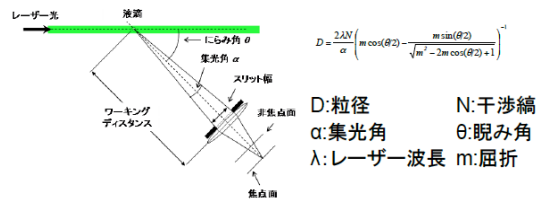
図3 ILIDSの原理
