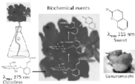
図7 デルフィニウムの花への香りの前駆体投与によるサクラモチの香り:クマリンの発散概念
