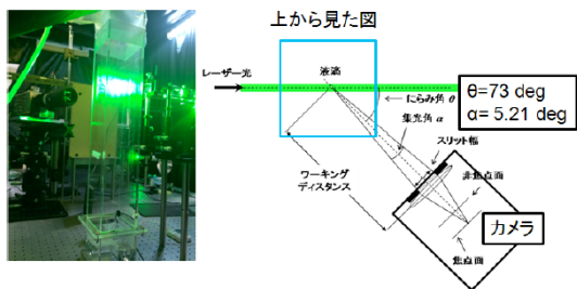
図4 装置の実際
