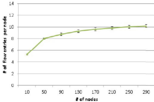
図3：ネットワーク規模とフローエントリ数
