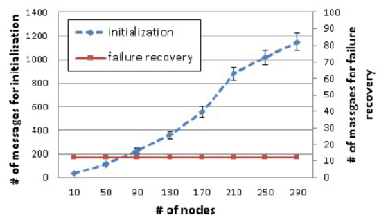
図 2：ネットワーク規模とメッセージ数
