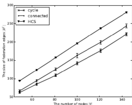
図5：ネットワーク規模とフェデレーショングラフのリンク数（NWS ランダムグラフ）
